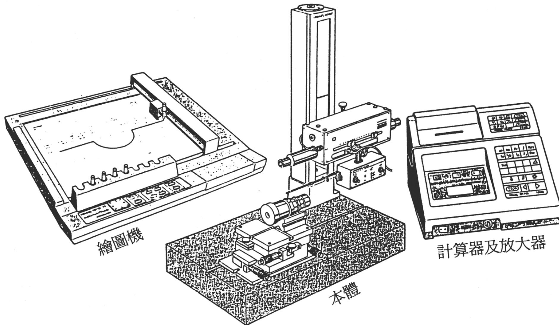
圖 6-3-1 輪廓量測儀 ( 德國 Hommel 公司出品，志邁科技公 司提供 )
