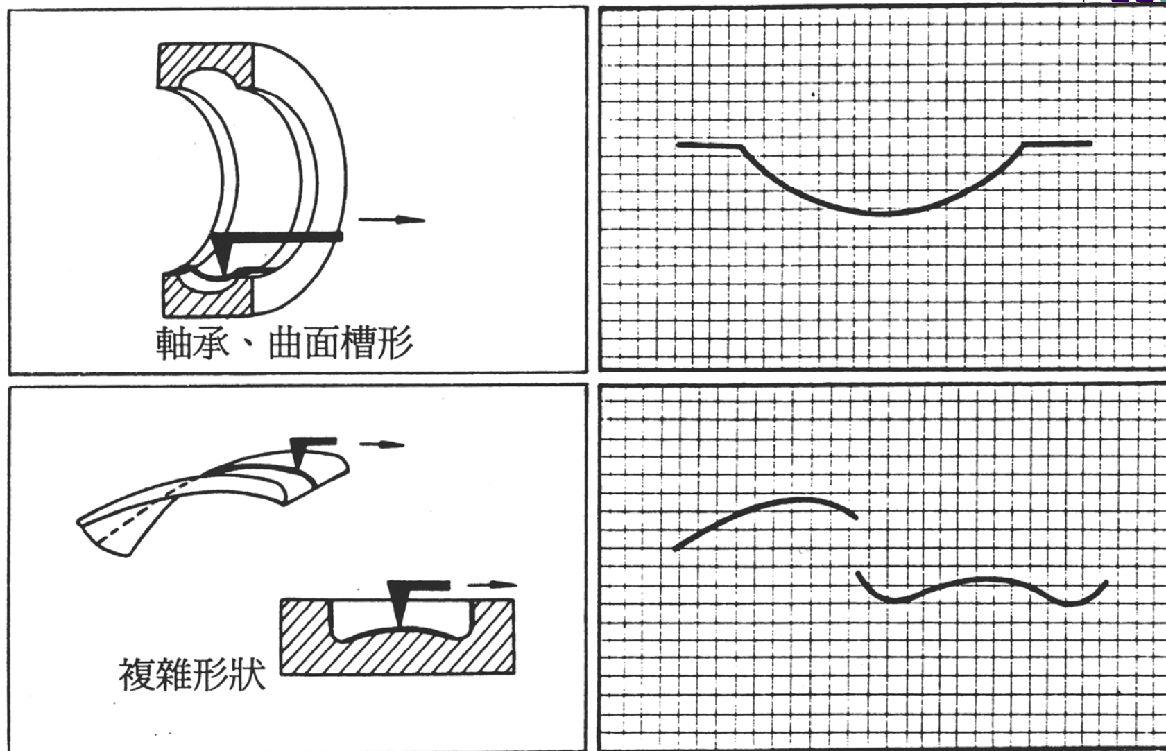
圖 6-3-5 輪廓量測工件實例 ( [25] )
