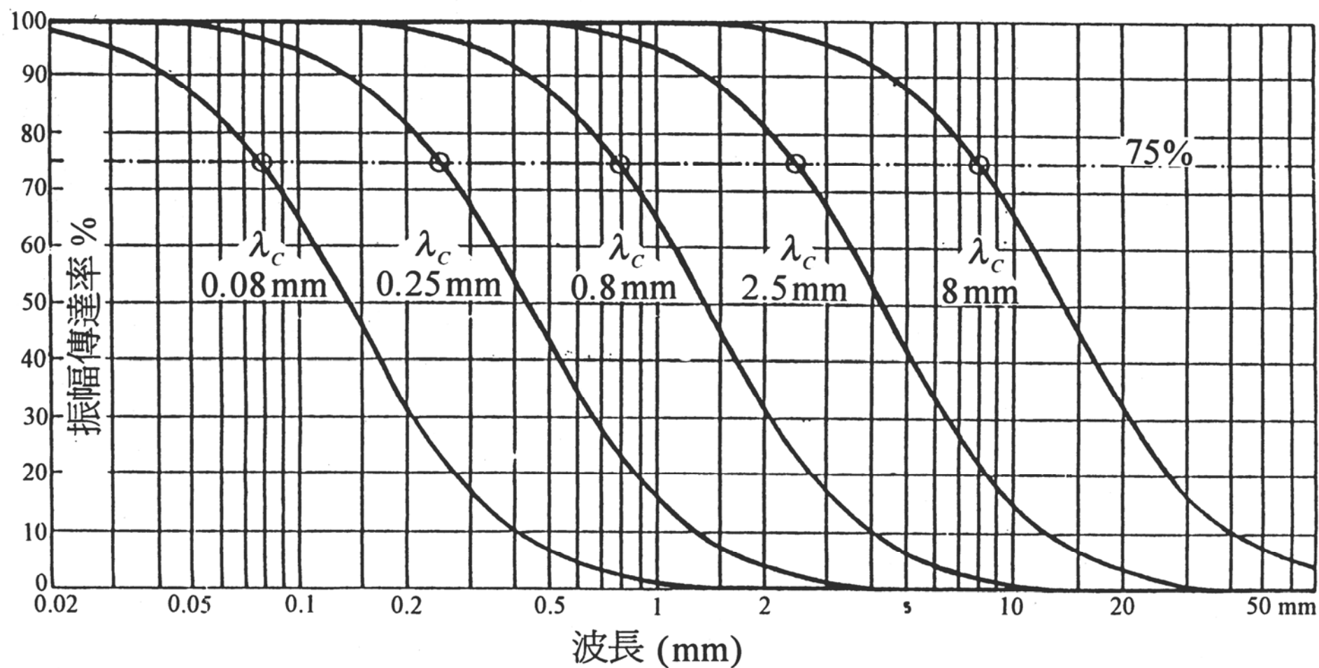
圖 6-1-1 輪廓之濾波特性圖 ( 德國 Mahr 公司操作手冊 , NO, 6800032 , P29 )
