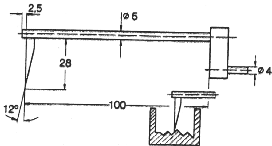
(a) 直支臂
