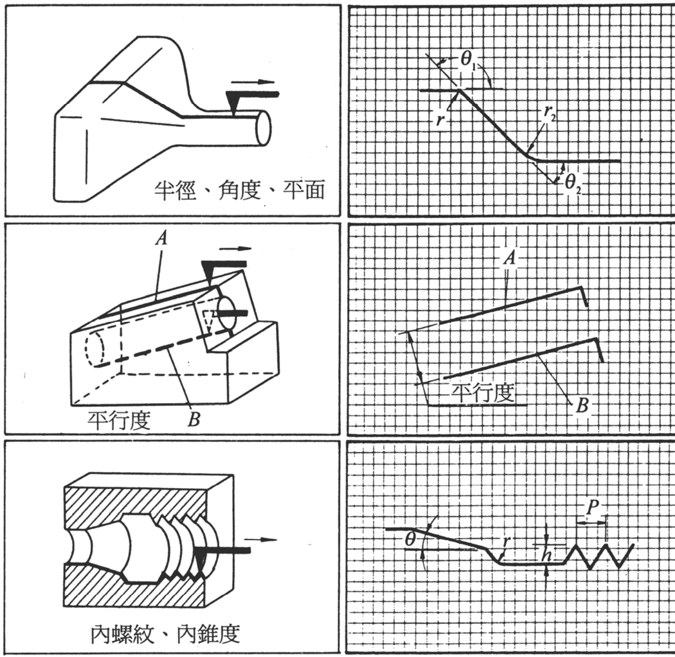
圖 6-3-5 輪廓量測工件實例 ([25])
