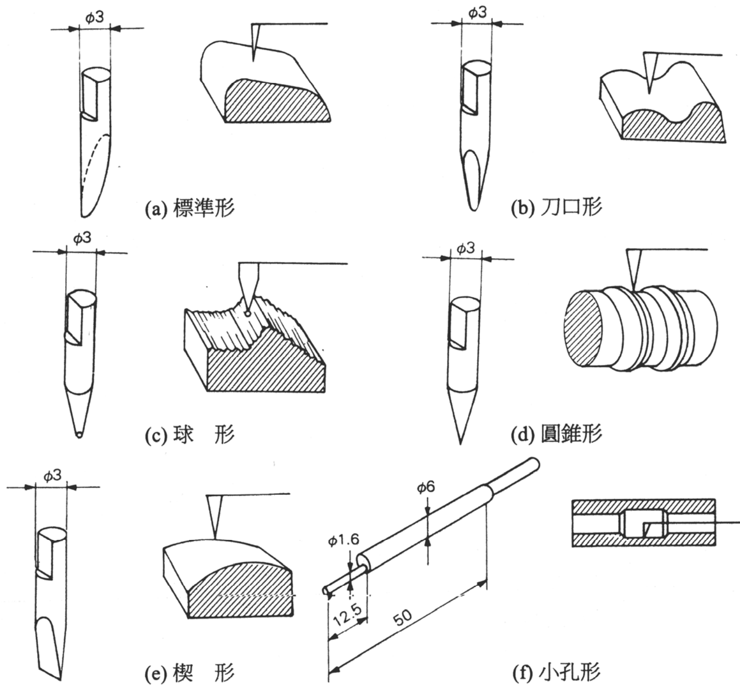
圖 6-3-3 探針之針尖形狀 ([22])
