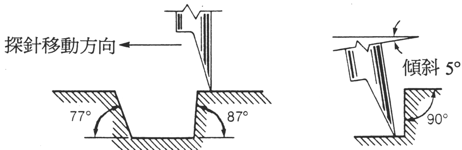
圖 6-3-4 探針運動方向與工件角度之關係
