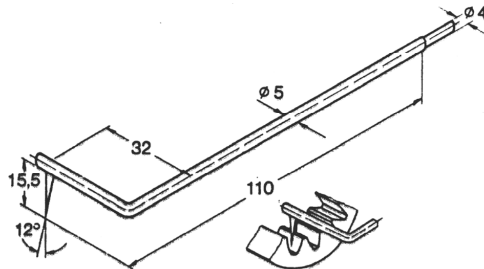
(b) 偏位支臂
